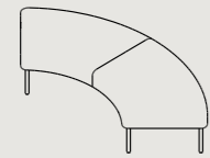
ASO90 W 1480 D 1480 H 440 IR 800
