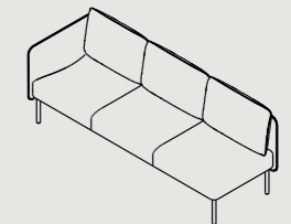
ASA3-R/L* W 2090 D 730 H 815 S 440
