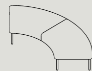
ASO90 W 1480 D 1480 H 440 IR 800
