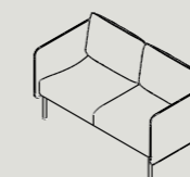
ASL2 W 1460 D 730 H 815 S 440
