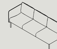
ASA3-R* W 2090 D 730 H 815 S 440
