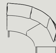
ASB90 W 1530 D 1530 H 815 S 440
