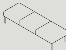
ASO3 W 2040 D 680 H 440
