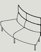
AMB60-R W 1610 D 1315 H 1025 S 440 IR 1200
