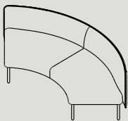
AB90 W 1530 D 1530 H 700 S 440 IR 800
