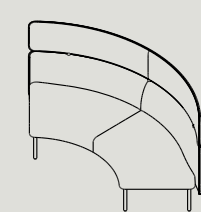
AMB90 W 1530 D 1530 H 1025 S 440 IR 800
