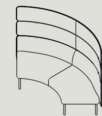
AHB90-D W 1530 D 1530 H 1350 S 440 IR 800
