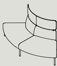
AMB90-R W 1480 D 1480 H 1025 S 440 IR 800
