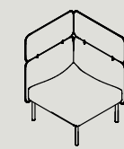
AMC1-R/L*^ W 730 D 730 H 1025 S 440
