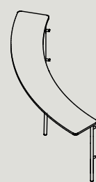
AD60-720 W 2200 D 570 H 720
