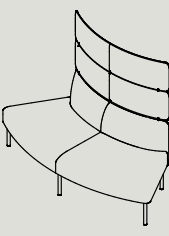
AB60-R-D W 1610 D 1285 H 1315 S 440 IR 1200
