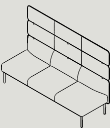
AMB3-D# W 2040 D 730 H 1350 S 440
