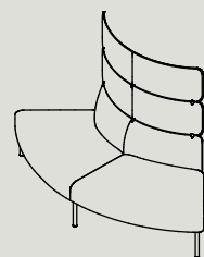
AHB90-R-D W 1480 D 1480 H 1350 S 440 IR 800
