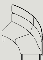
AMB60 W 1660 D 1315 H 1025 S 440 IR 1200
